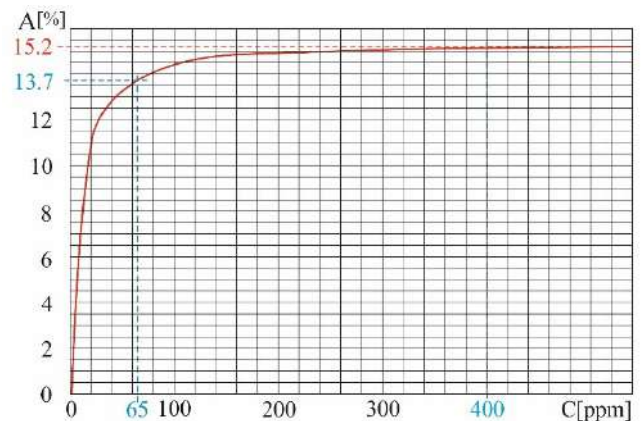
Wykres 3. Zależność absorpcji ziemskiego promieniowania cieplnego w atmosferze od stężenia CO 2
