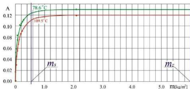
Wykres 2. Zależność między absorpcją przepuszczanego promieniowania cieplnego a masą CO 2
