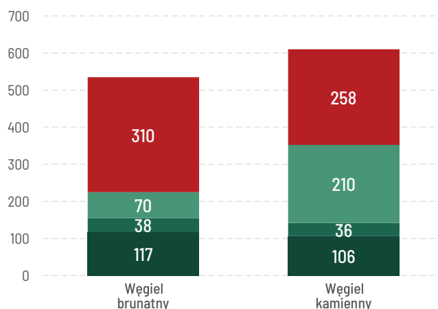
Wykres 3. Koszty produkcji energii elektrycznej z węgla brunatnego i kamiennego (w PLN/MWh)
